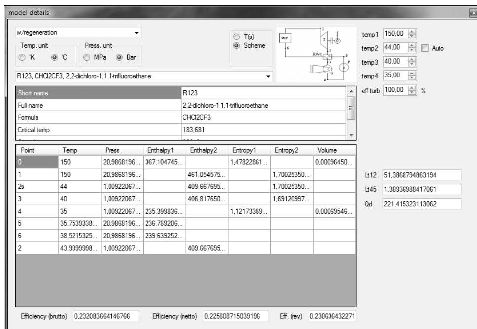
Rys. 4. Parametry termodynamiczne w punktach charakterystycznych układu Fig. 4. Thermodynamic parameters of the system's characteristic points
